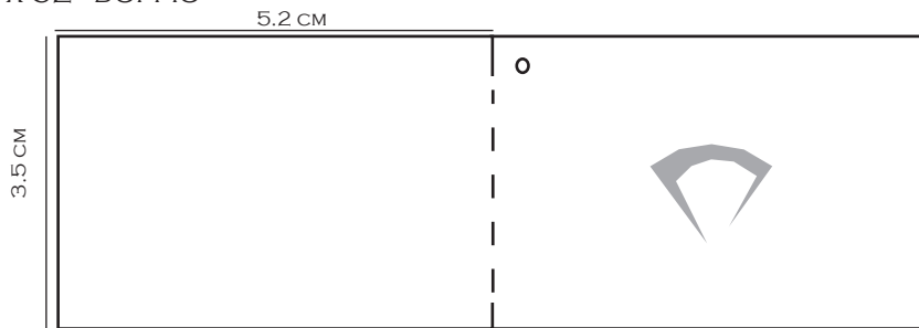
FUSTELLA N°24 35 X 52 - DOPPIO
